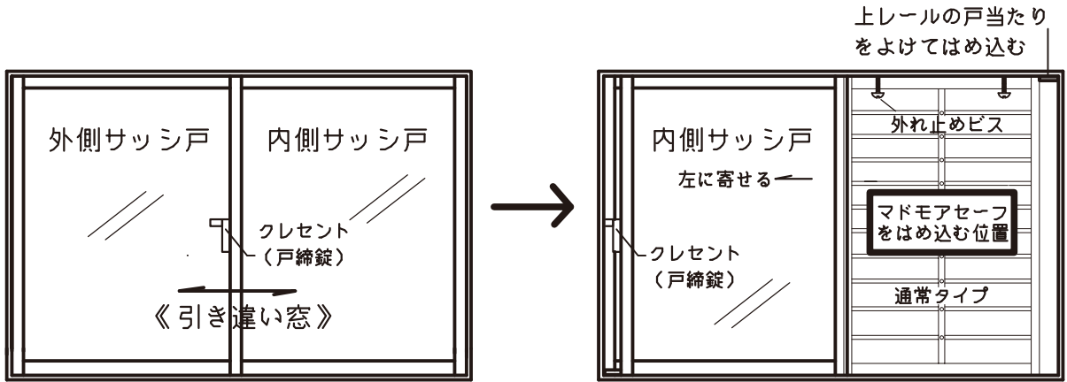
窓を室内から見た正面図
