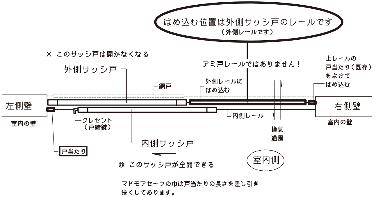
窓を真上から見た平面図
