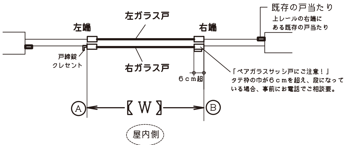
—— 断面図 ——
