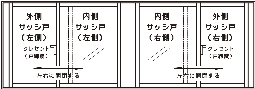
4連引き違い窓
